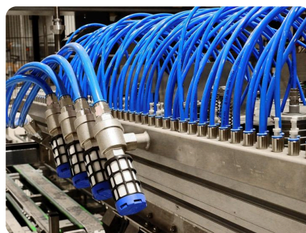
Vanne pneumatique INSTALLATION MÉCANIQUE
