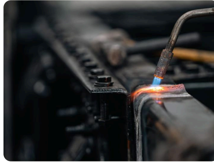
Kaynak kordonu
