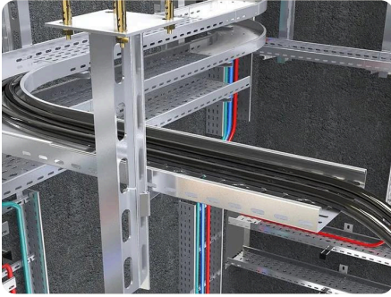
Kablo kanalı ve kapağı
